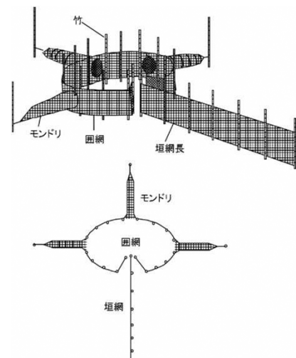
定置網の構造
