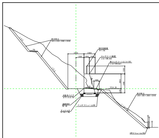
標準断面図
