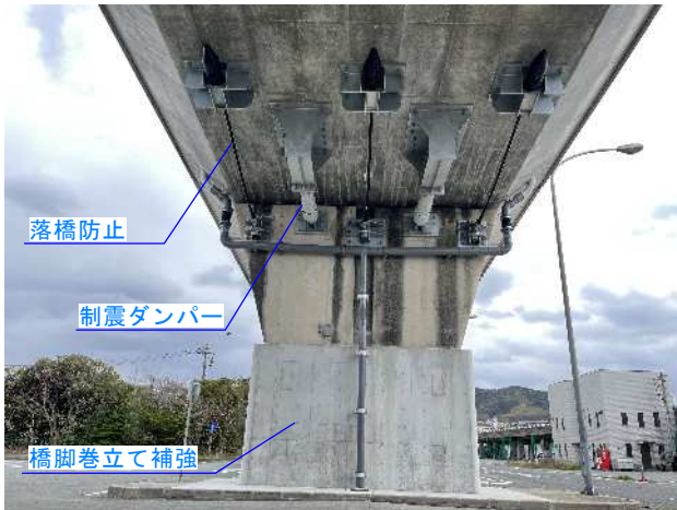
P 5 橋脚
