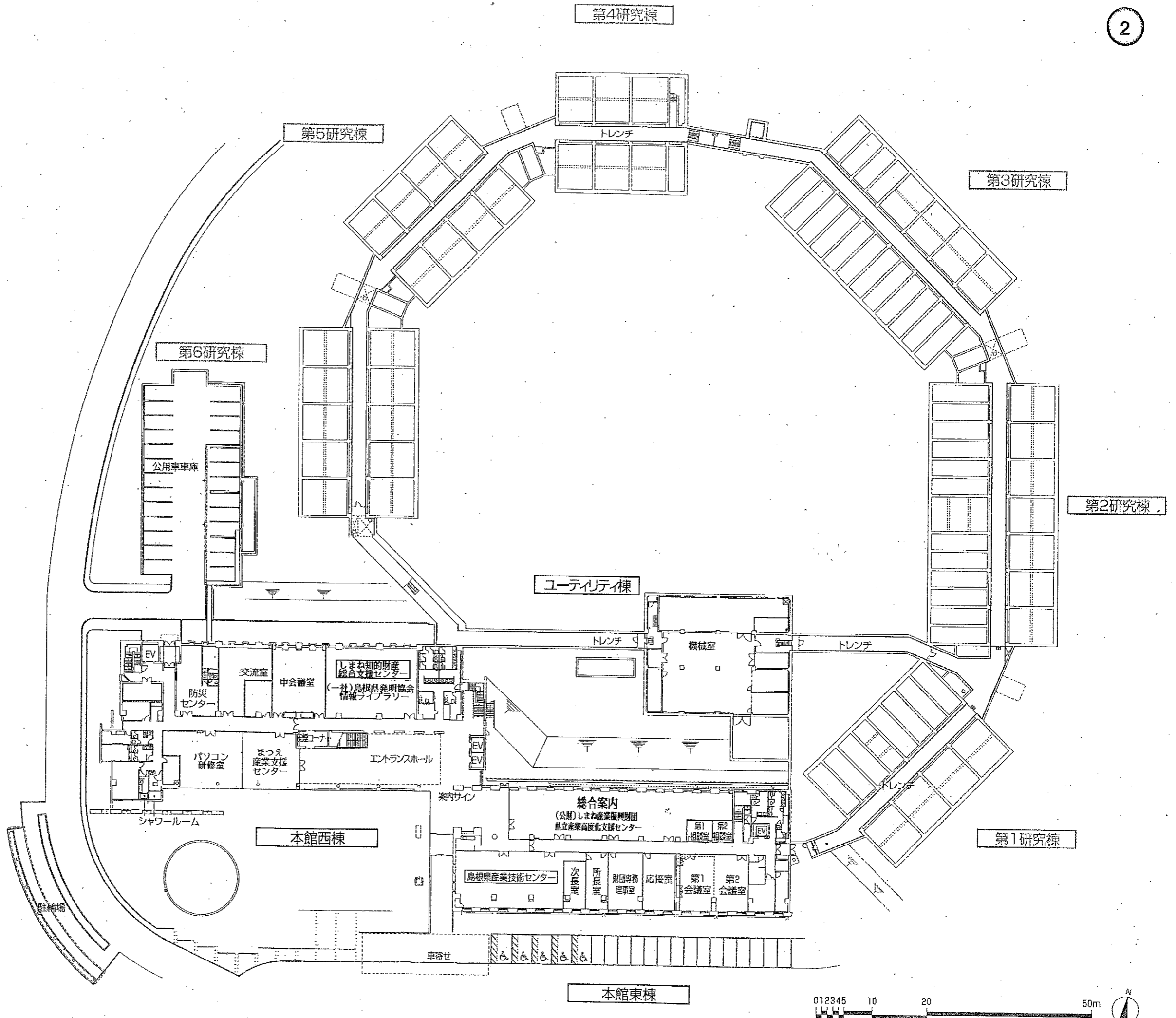
1F平面図
