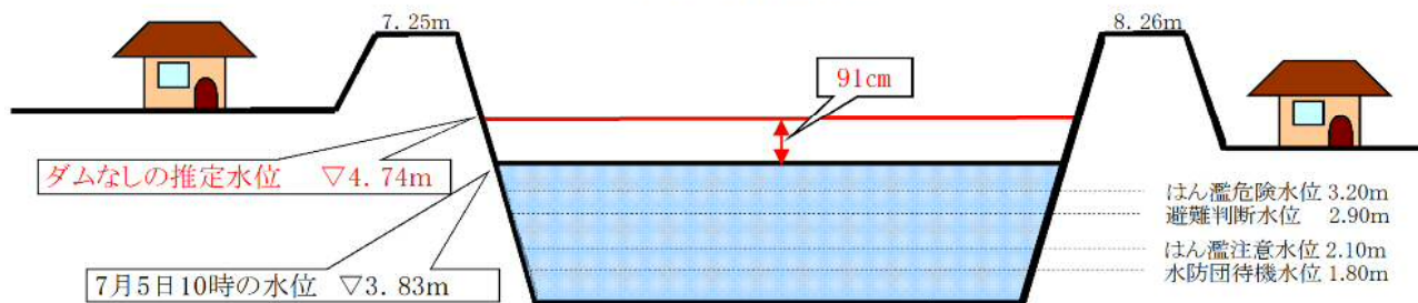
中場水位局付近断面図 (島根県浜田市穂出町)
