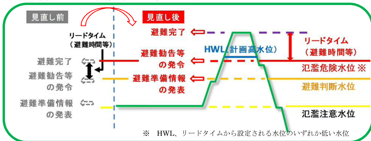
危険箇所設定断面図（飯梨川、周布川、益田川等）
