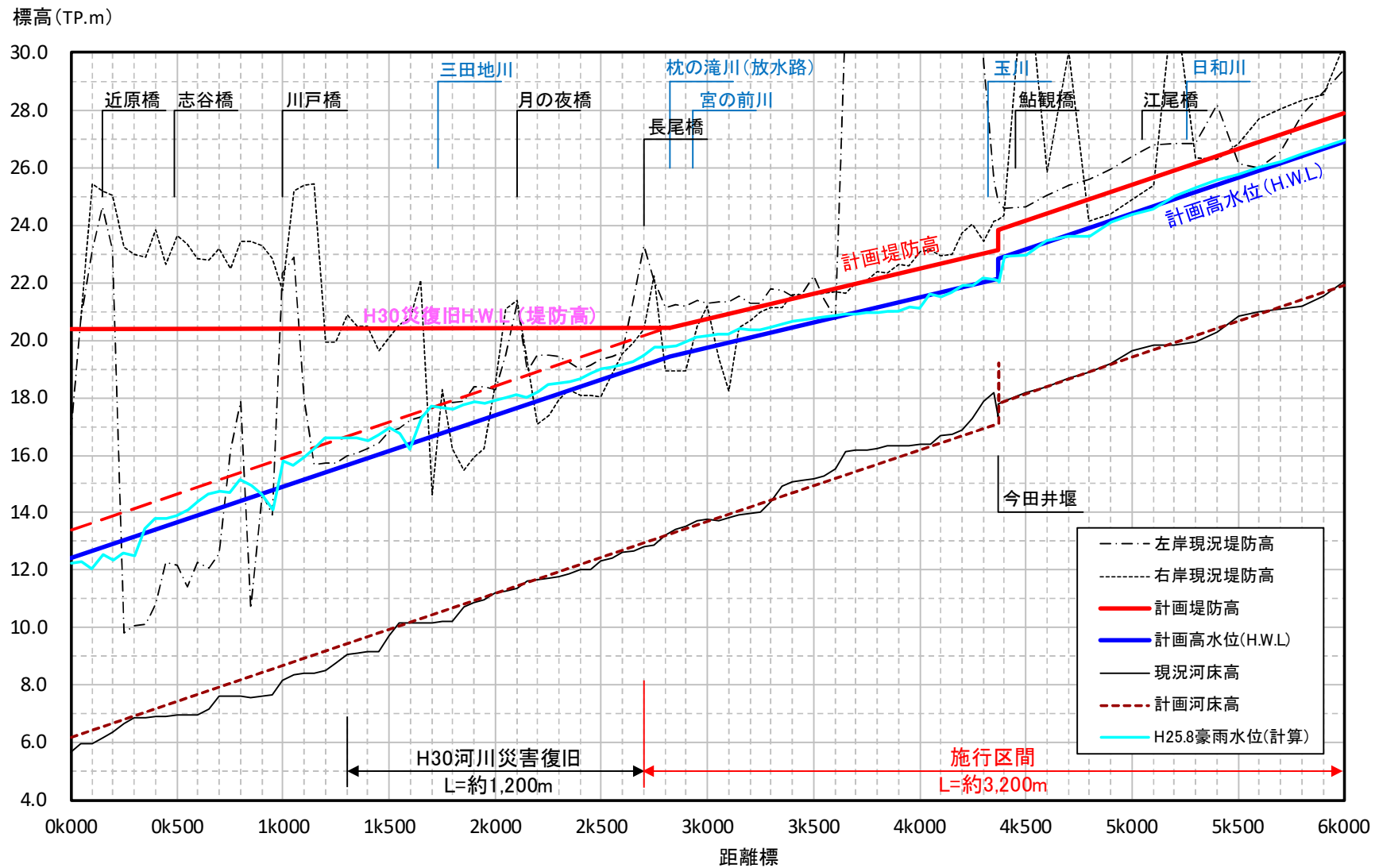
図-4.1.5 河道の縦断形 (八戸川)
