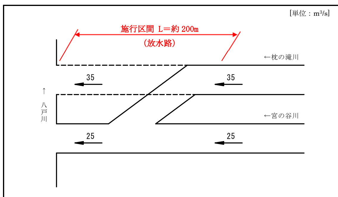
図-4.1.7 整備計画目標流量図（枕の滝川）
