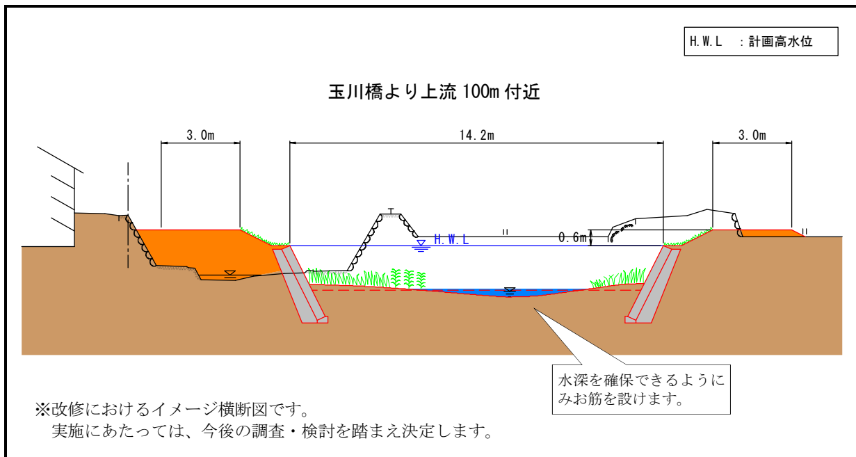
図-4.1.12 河道の横断形 (玉川) (S=1/200)
