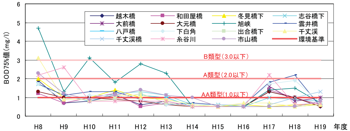
図-3.3.1 BOD (生物化学的酸素要求量) の推移
