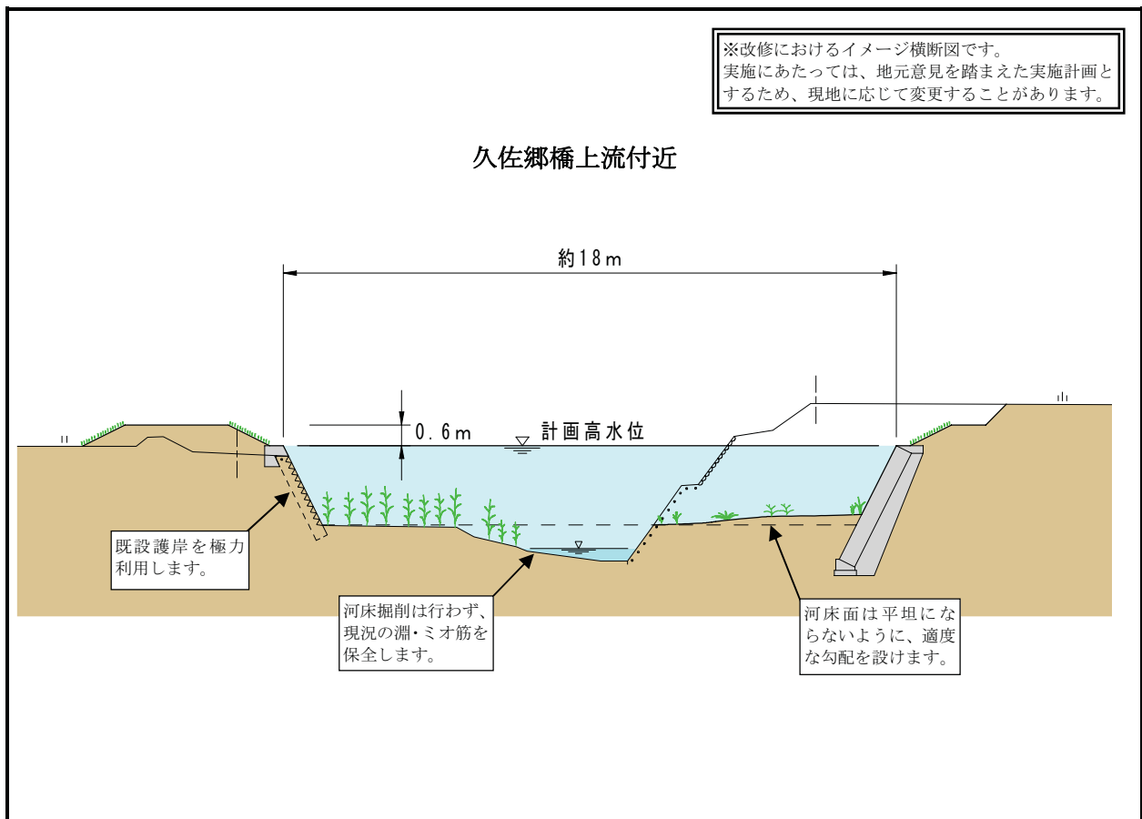
図-4.1.4 河道の横断面形 (S=1/200)
