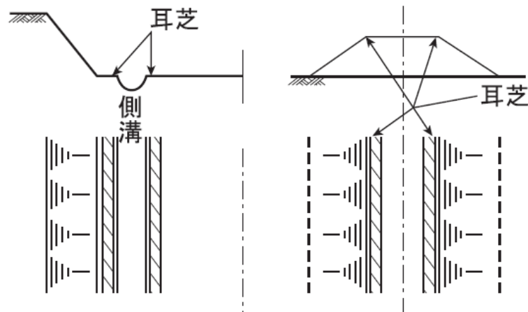
図 3-2-6 耳芝
