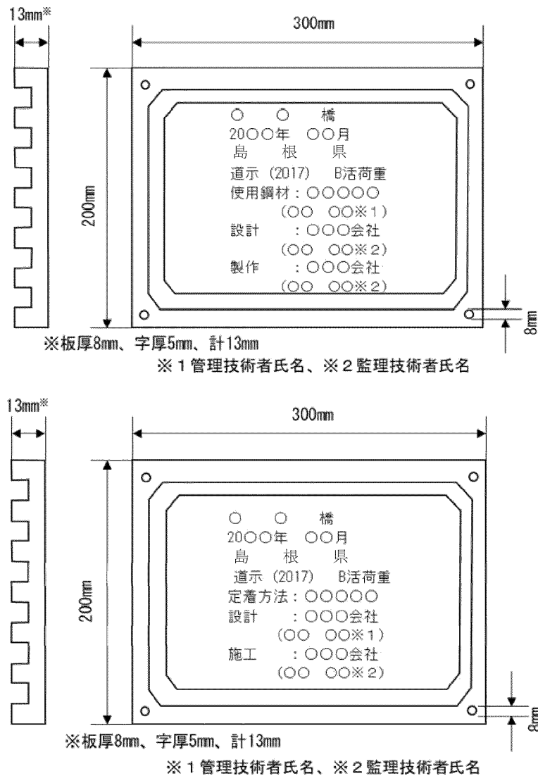
図 3-2-2 銘板の寸法及び記載事項
