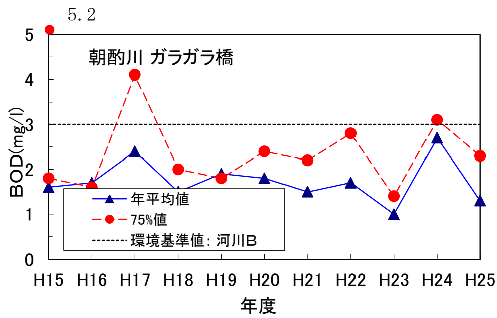
図8 松江市内河川のBODの経年変化
