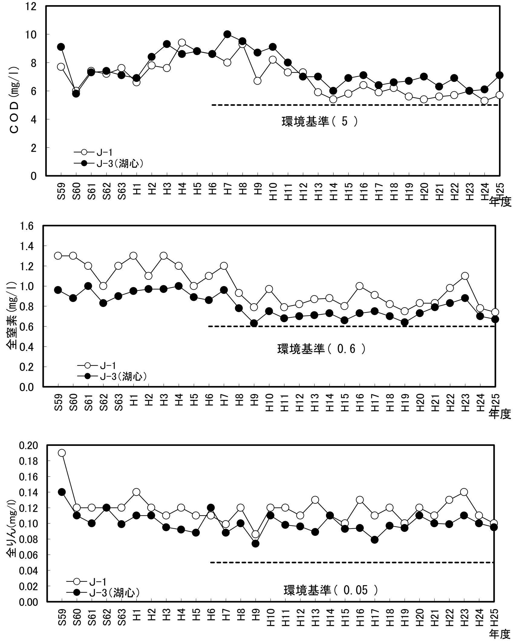
図 1 2 神西湖の環境基準点におけるCOD、T-N、T-Pの経年変化
