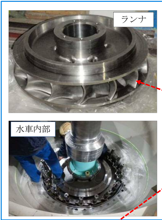
水車 (地下2F)
