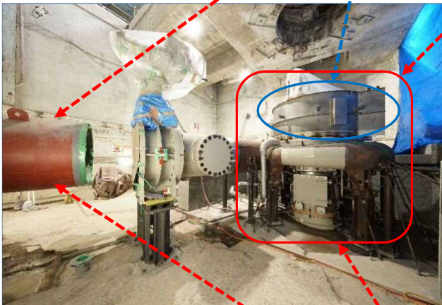
水圧鉄管・水車外部・入口弁 (地下3F)
