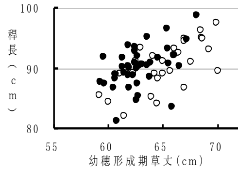
第8-3図 「コシヒカリ」における幼穂形成期の草丈と稈長の関係(5月下旬植, 島根農試) ○2000年 ●2001年
