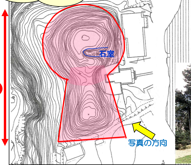
平神社古墳の測量図
