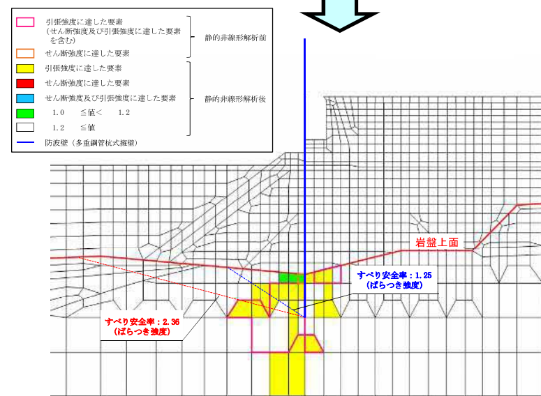
図4 岩盤の局所安全係数分布図 (③-③断面, 静的非線形解析後)
