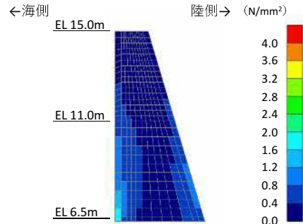
図15 コンクリートの最大せん断応力図
