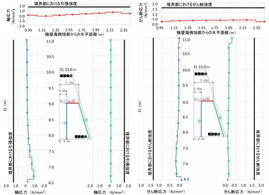
図17 境界部における引張応力図
