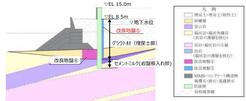
図2 断面図（②-②断面）
