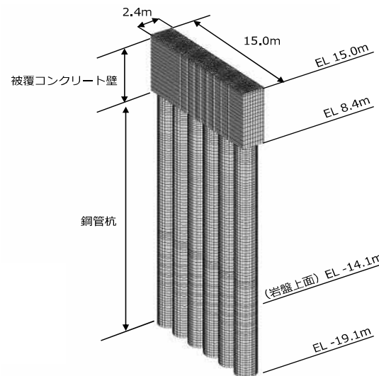
図7 評価対象位置（②-②断面）
