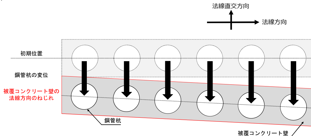
図2 被覆コンクリート壁のねじれの概念図
