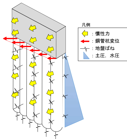
図5 3次元静的FEM解析への荷重入力イメージ
