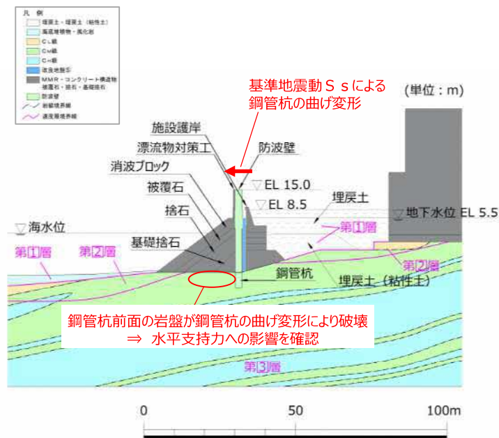
図2 断面図 (③-③断面)
