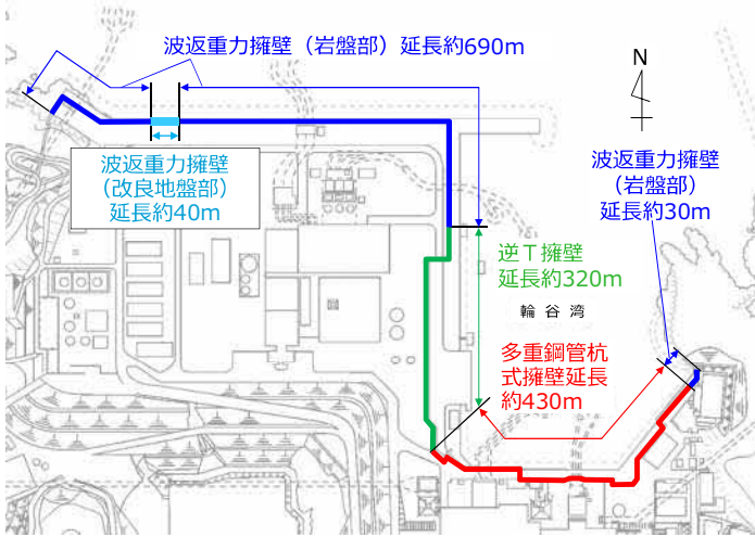
図 1 防波壁の位置図
