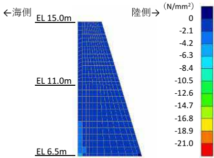
図14 コンクリートの最小主応力図
