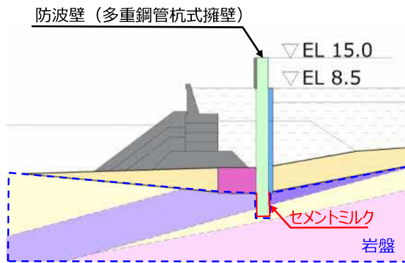
図8 解析モデル図
