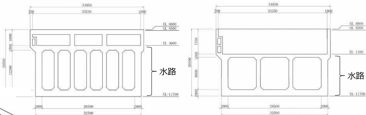
(A-A断面)
