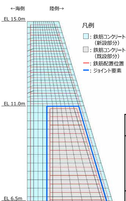
図12 解析モデル図
