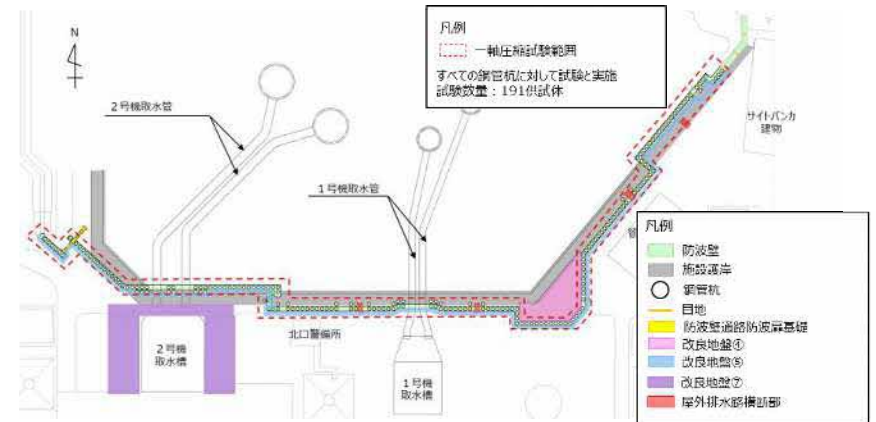
図9 セメントミルクの一軸圧縮試験範囲
