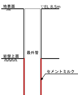
図7 セメントミルクの配置図
