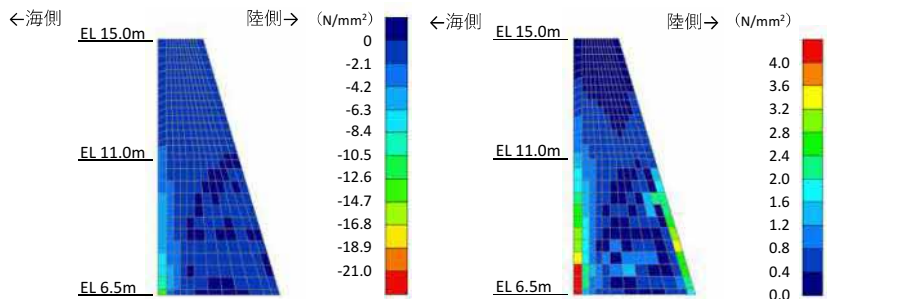
図20 コンクリートの最小主応力図 図21 コンクリートの最大せん断応力図
