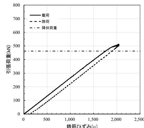
図10 実験結果（引張荷重－鉄筋ひずみ関係） （鉄筋D41）
