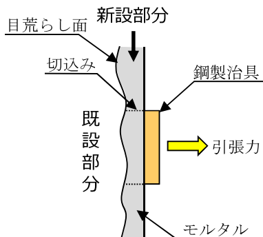
図4 付着強度試験イメージ
