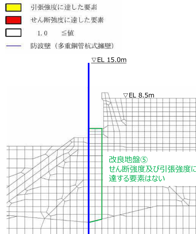
図6 改良地盤⑤の破壊履歴図（例：③－③断面）
