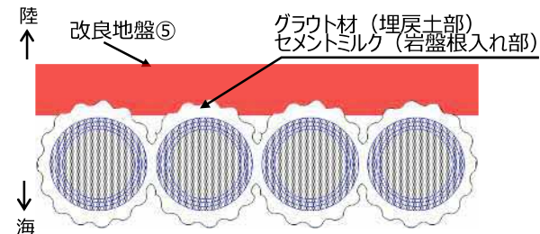
図3 地中断面図
