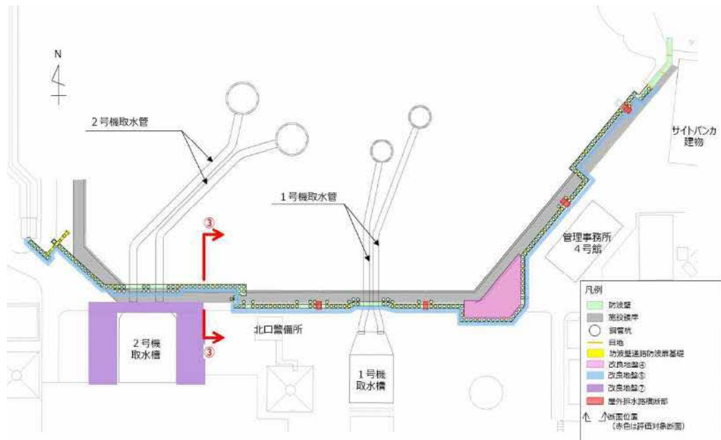
図1 平面図
