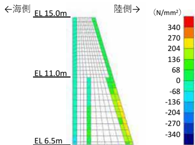
図22 鉄筋の応力図
