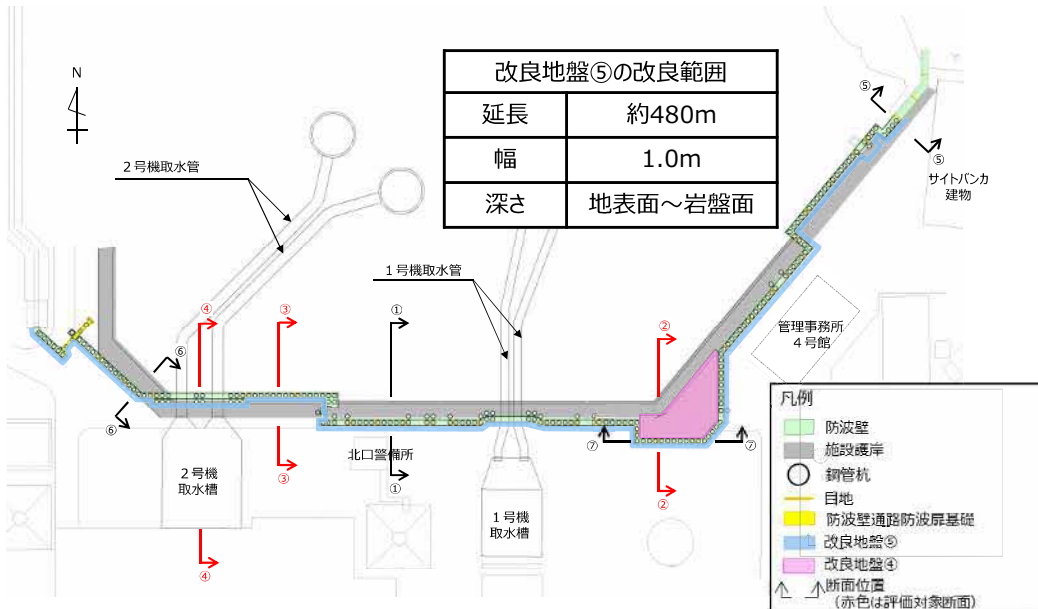
図1 平面図
