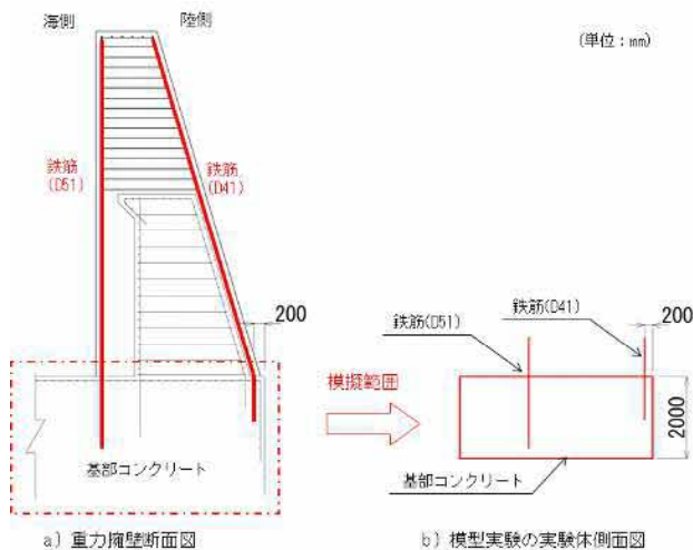
図7 重力擁壁の実験体における模擬範囲
