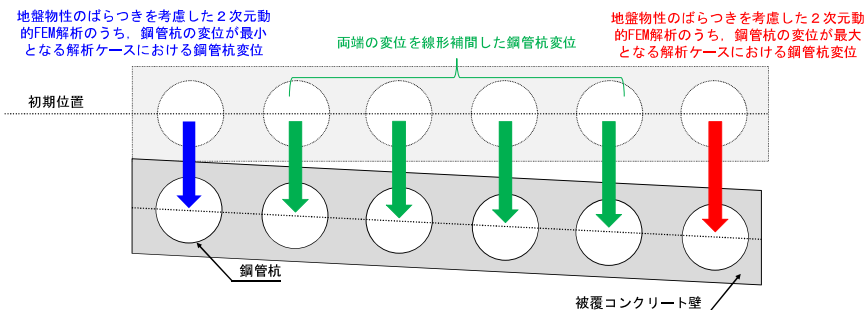
図4 鋼管杭変位の入力イメージ
