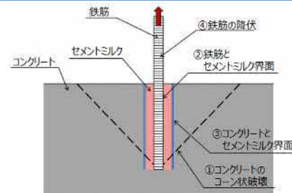
図9 想定される破壊形態
