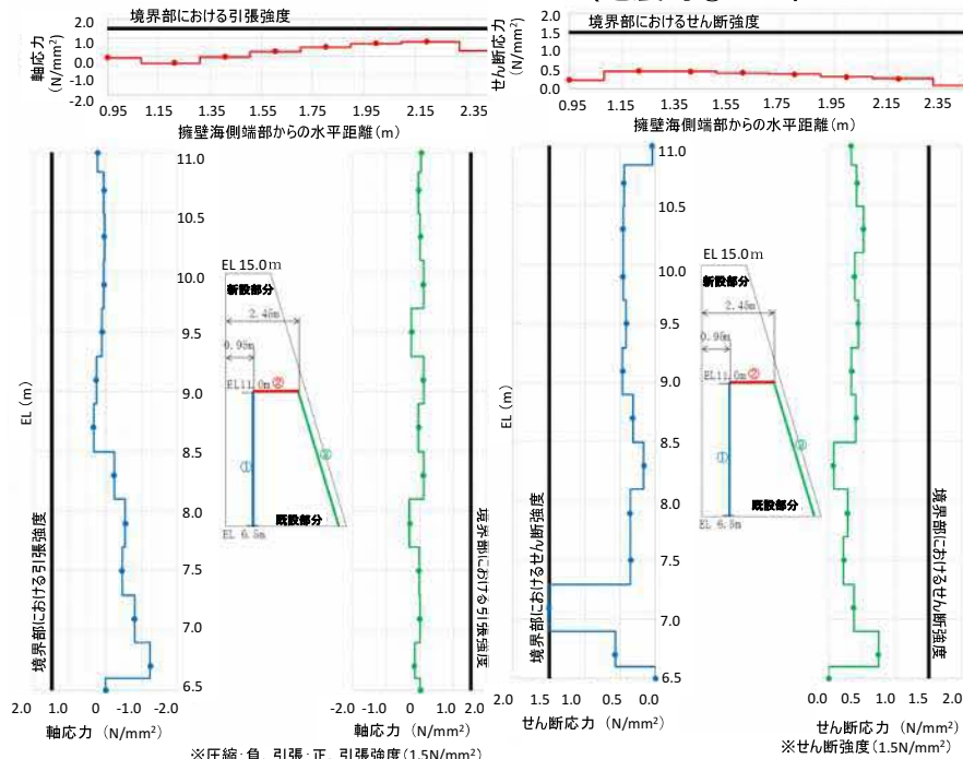
図23 境界部における引張応力図 図24 境界部におけるせん断応力図
