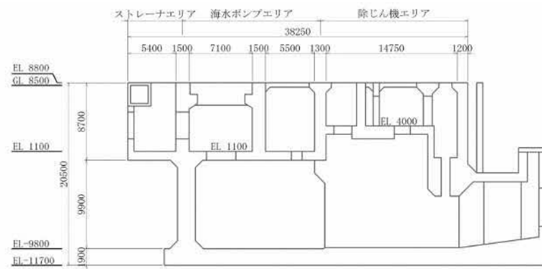
(D-D断面)
