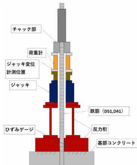
図8 載荷装置及び計測位置概要図
