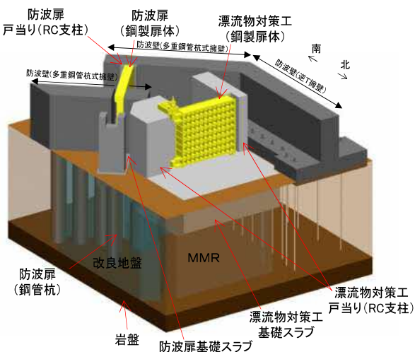
図7 防波扉（荷揚場南）の構造概要図
