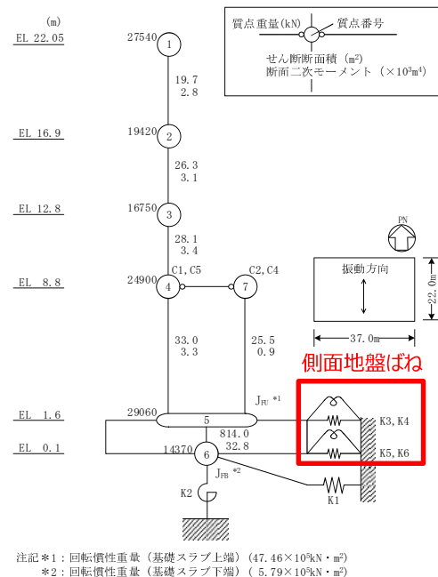
図13 側面地盤ばね考慮モデル (NS方向)
