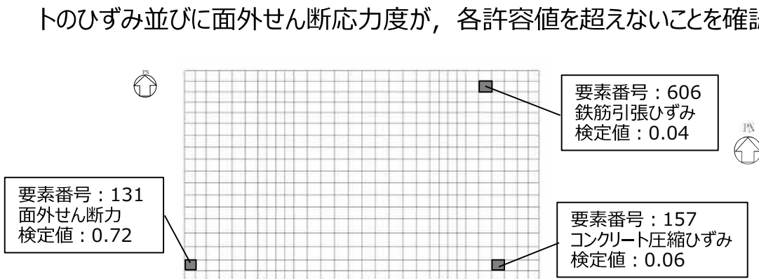
図11 断面力ごとの検定値が最大となる要素及び断面の評価結果
