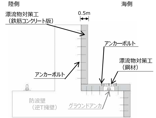
図1 防波壁に設置する漂流物対策工
