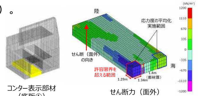
図9 発生応力コンター図 (③-③断面、底板①、せん断(面外))
