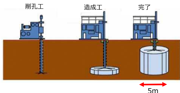
図 3 高圧噴射攪拌工法の施工イメージ
