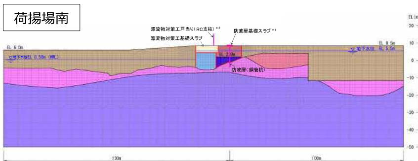
図5 2次元解析モデル図 (荷揚場南)
