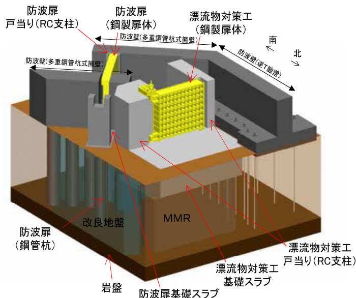
図2 防波扉（荷揚場南）の構造概要図
