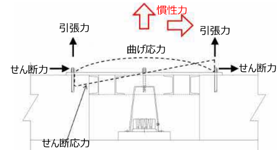
図7 各部位に生じる発生力等のイメージ図
