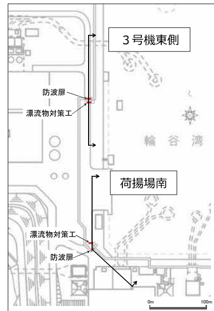
図4 評価対象断面位置図
