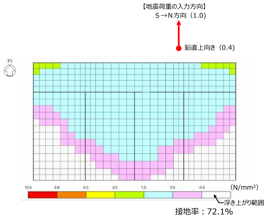
図10 接地圧分布
