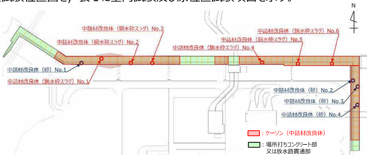
図 5 原位置試験（PS検層）位置図
