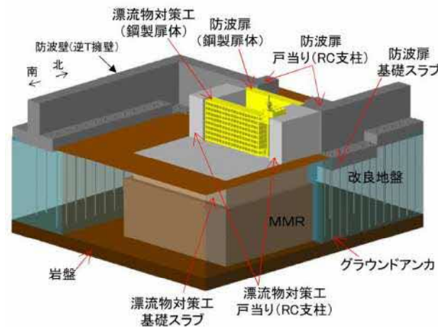
図8 防波扉（3号機東側）の構造概要図
