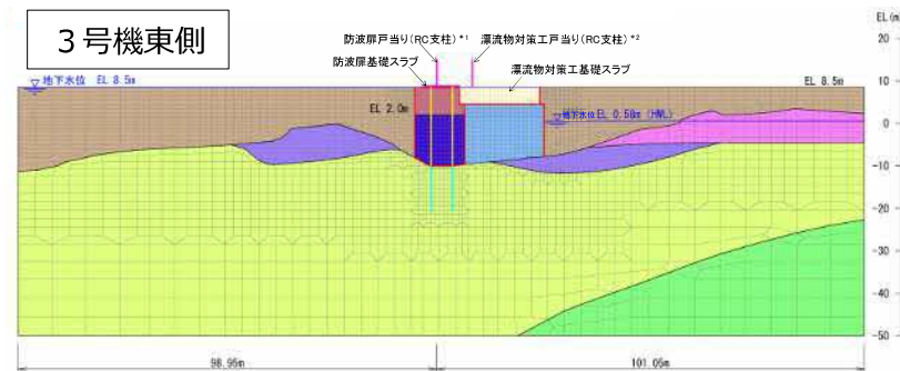
図6 2次元解析モデル図 (3号機東側)
