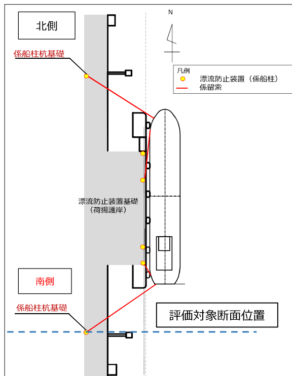
図1 係船柱杭基礎の設置位置
